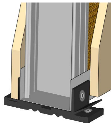
Εφαρμογή Vibro-WS σε πλωτό χώρισμα από γυψοσανίδα
