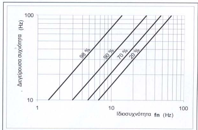
3. ΔΙΑΓΡΑΜΜΑ ΘΕΩΡΗΤΙΚΗΣ ΜΕΙΩΣΗΣ ΚΡΑΔΑΣΜΩΝ
